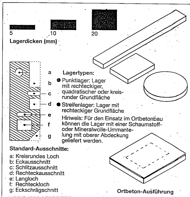
Abbildung 1: Calenberg Kerncompactlager
