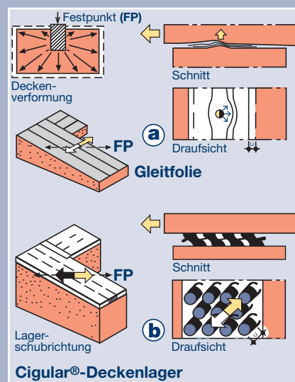
Bild 3: Funktionsprinzip einer Gleitfolie (a) und des Cigular®-Deckenlagers (b).
