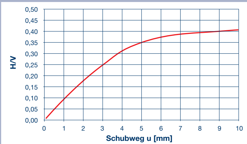
Bild 5: Verhältnis der Horizontalkraft zur Vertikalkraft
